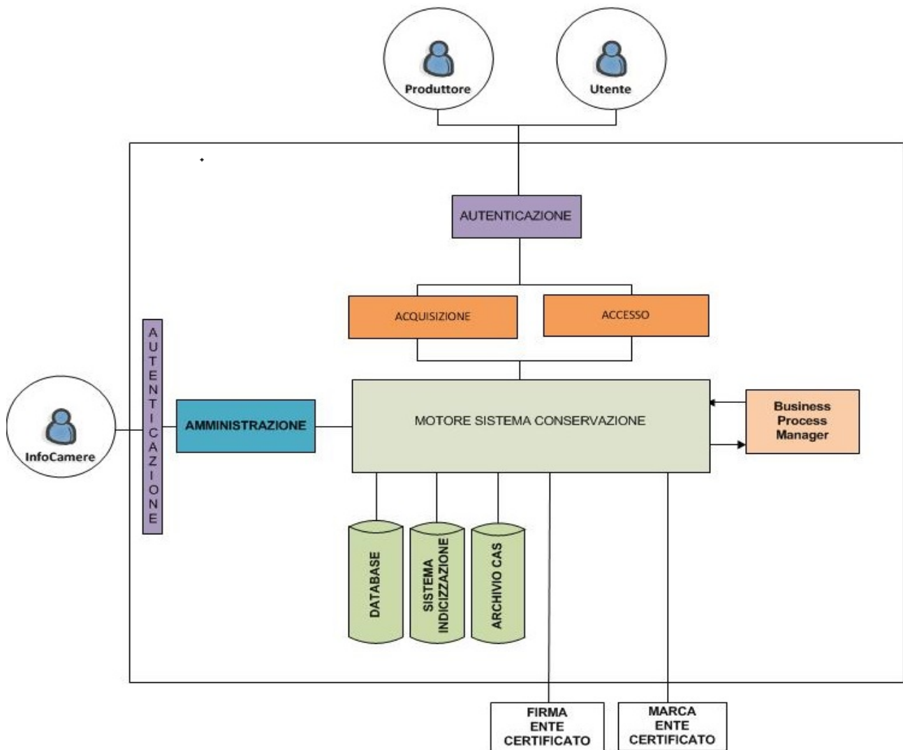
Figura 15 Schema componenti tecnologiche
