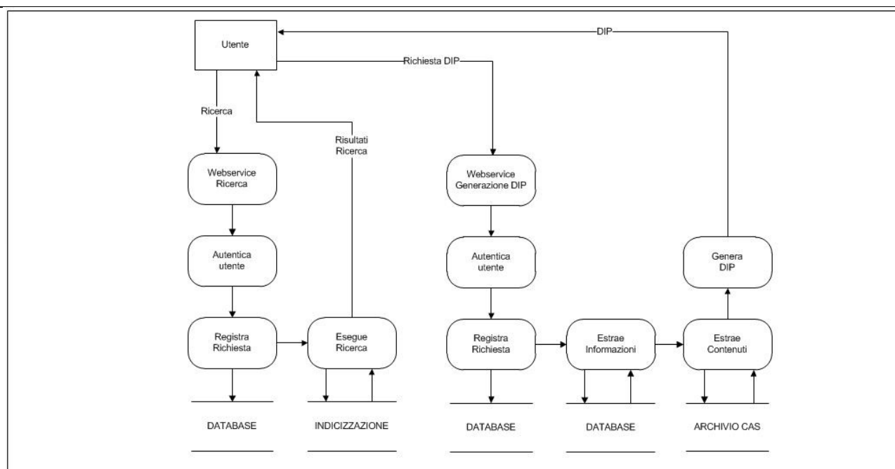
Figura 13 Generazione pacchetto di distribuzione
