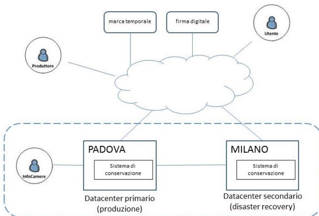
Figura 16 Schema dei siti di conservazione
